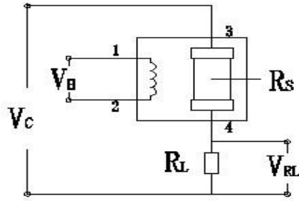
图2: WSP2110 测试电路
